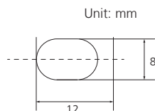
Befestigungsbohrung
