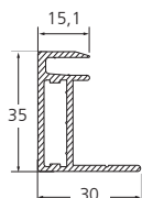
Rahmenquerschnitt
